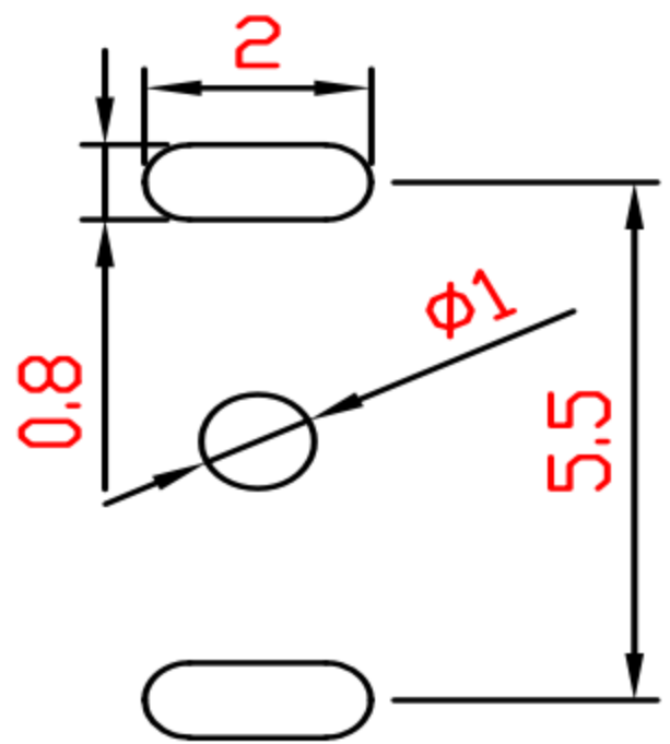
图为焊盘位置和大小
