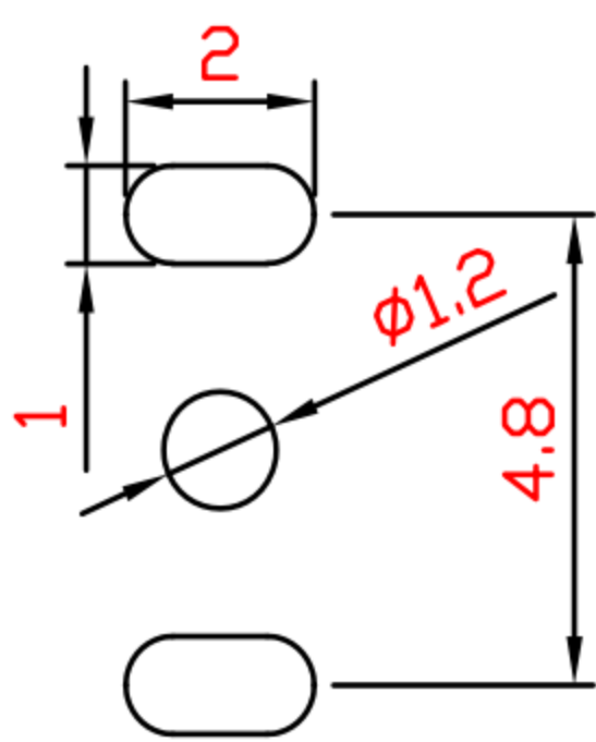
图为焊盘位置和大小
