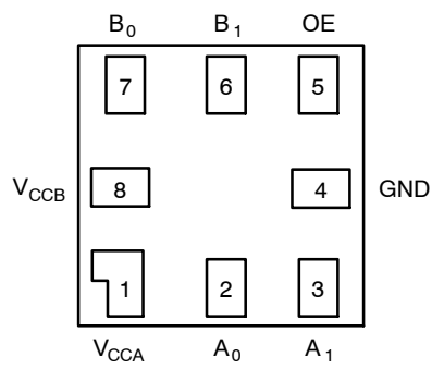
图 2. MicroPak（顶视图）
