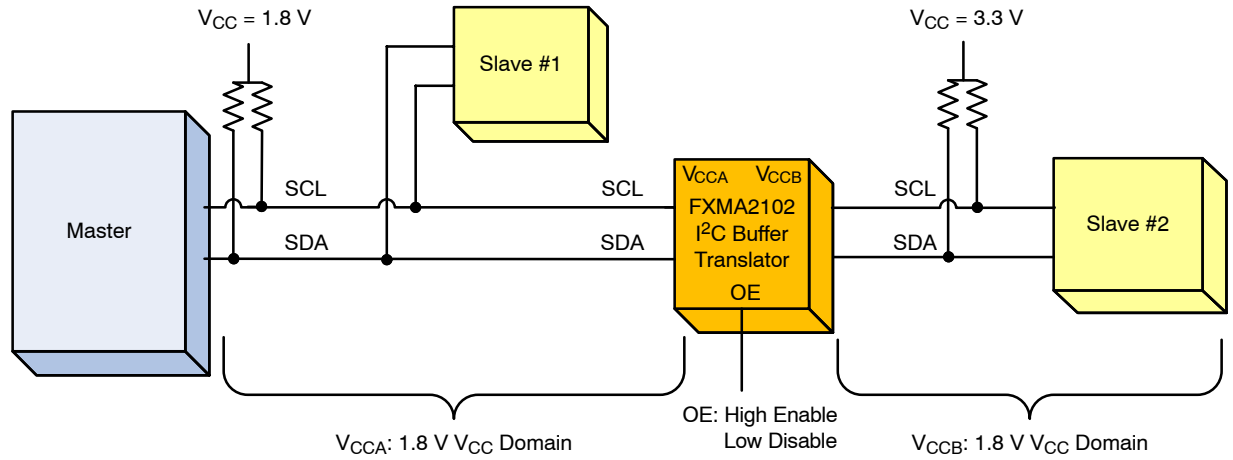
图 7. 总线隔离
