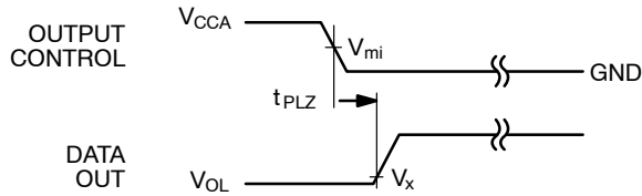
图 11. 3态输出高电平使能时间 (说明 15)
