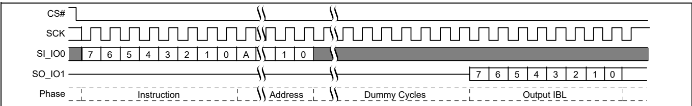
图 95 IBLRD 命令序列 [53、54]
