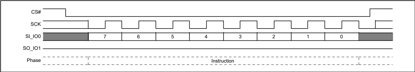
图 86 芯片擦除命令序列
