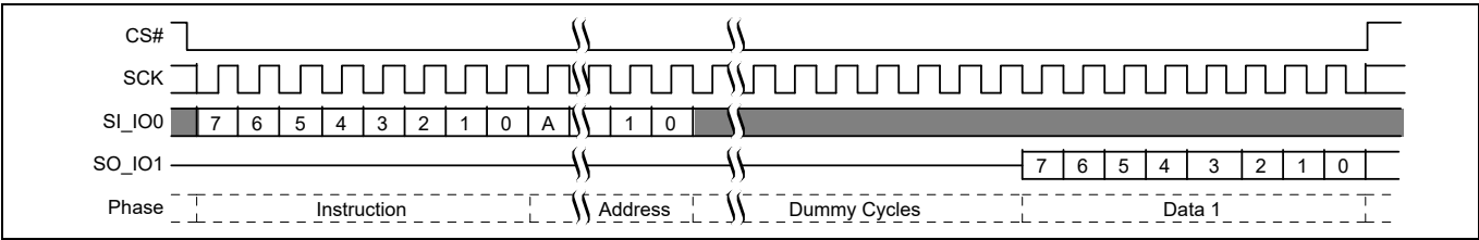
图 31 RSFDP 命令序列
