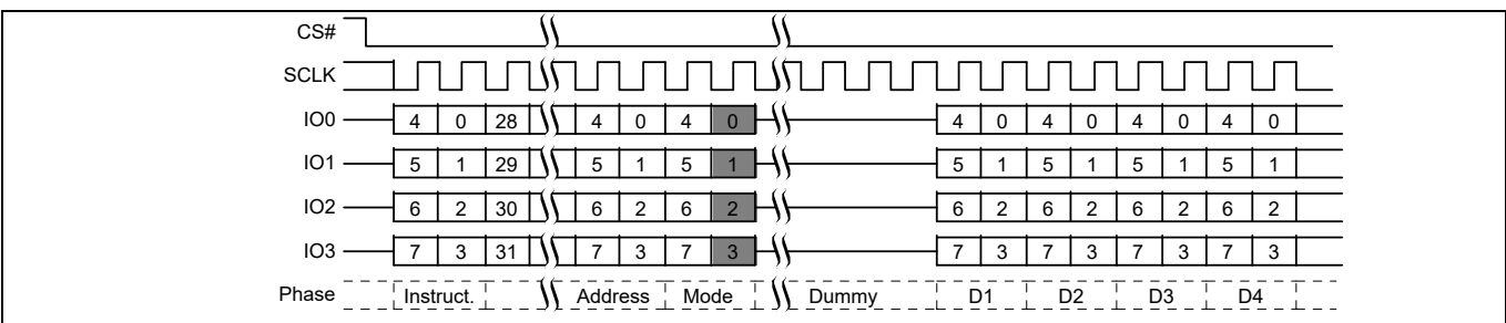
图 21 在 QPI 模式下的四线 I/O 读命令 [8]
