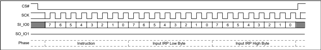
图 109 IRP 编程 (IRPP) 命令
