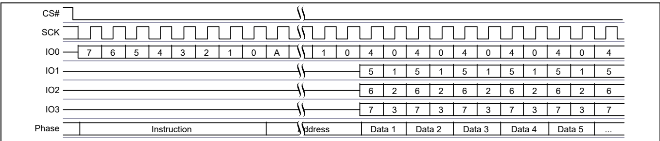
图 79 四线页编程命令序列 [45]
