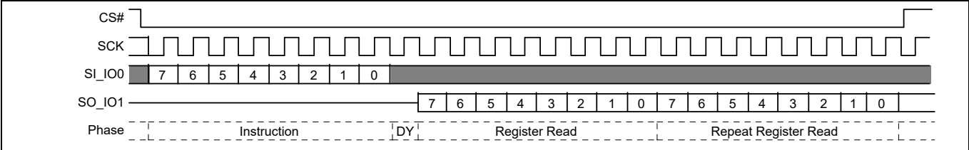
图 53 DLP 读取 (DLPRD) 命令序列
