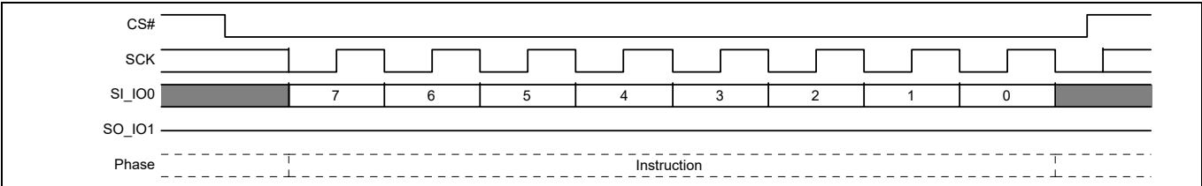
图 47 清除状态寄存器 (CLSR) 命令序列
