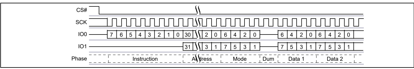
图 19 双线 I/O 命令
