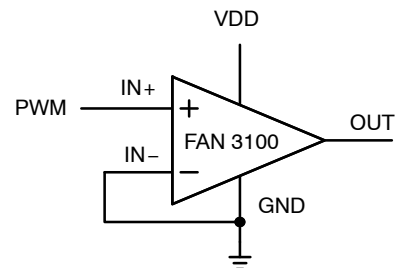
图 41. 使能的双输入驱动器，同相配置
