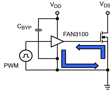
图 40. MOSFET 关断时的电流通路
